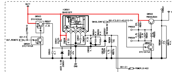
Batt SW
