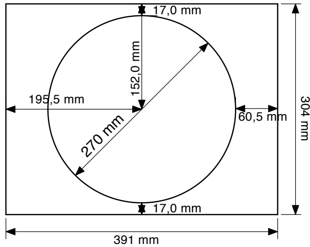
Лицевая панель
