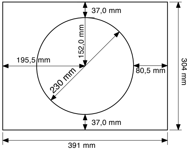
Передняя стенка
