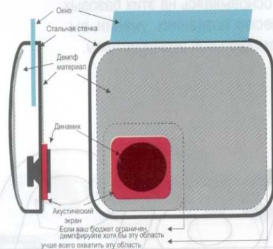
Схема подавления вибрации дверей
