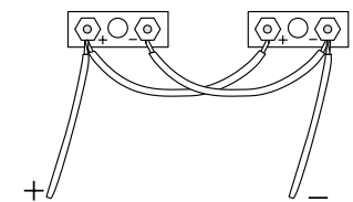
Afbeelding 2. Serie aansluiting
