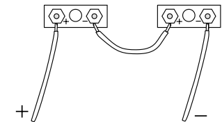
Figura 2. Conexión en serie.
