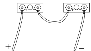
Afbeelding 2. Serie aansluiting
