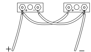
Figura 2. Conexión en serie.
