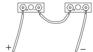
Figure 2. Raccordement en série.
