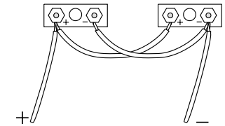
Figure 1. Raccordement en parallèle.
