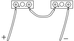
Abbildung 2. Serielle Verkabelung
