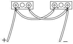
Abbildung 2. Serielle Verkabelung
